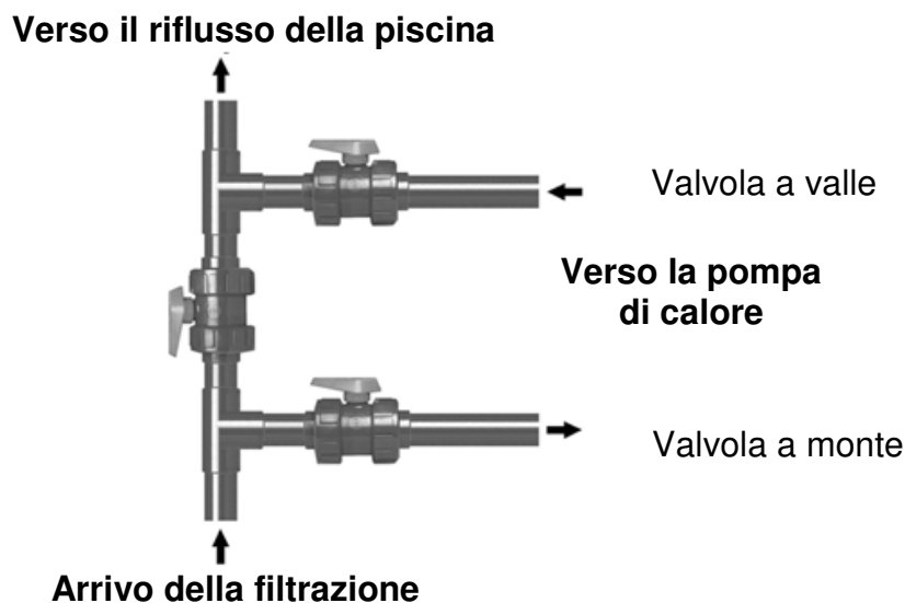
Schema del by-pass
