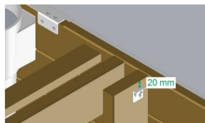
Figure 35 – Positionnement de la gâche de serrure
