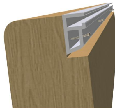
Figure 26 - Pose du rail d'accrochage
