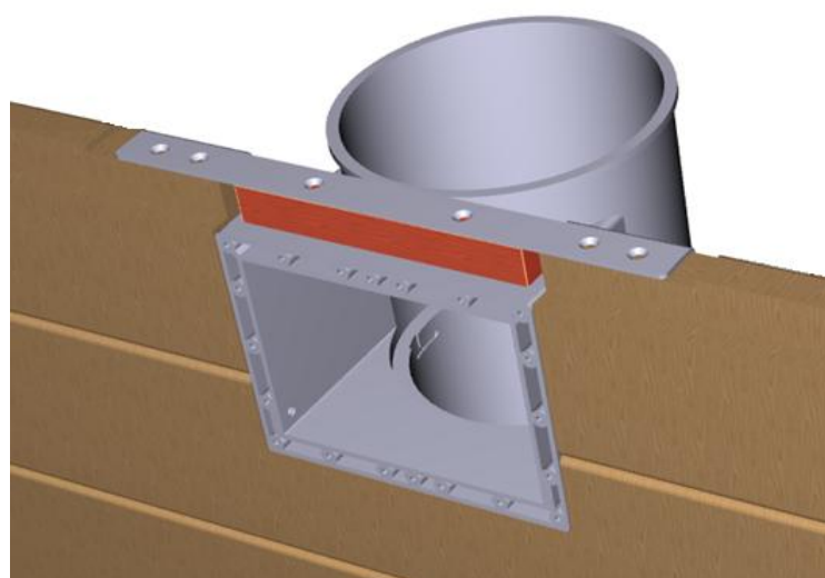
Figure 23 - Montage de l'équerre de skimmer
