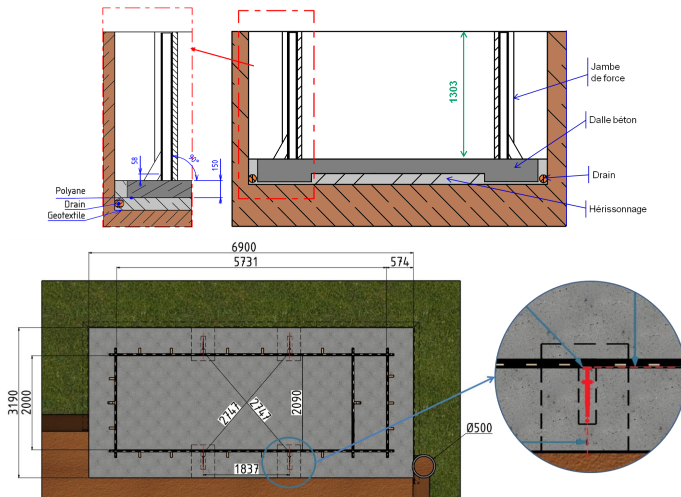
Figure 4 - Positionnement des jambes de force
