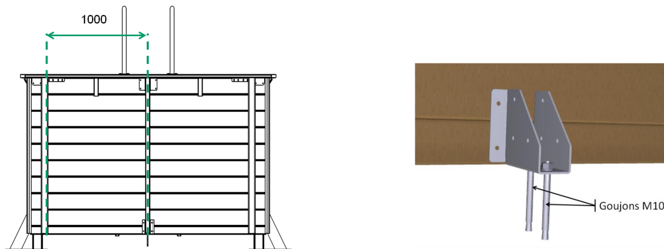
Figure 12 - Pose des sabots pour jambes de force en bois
