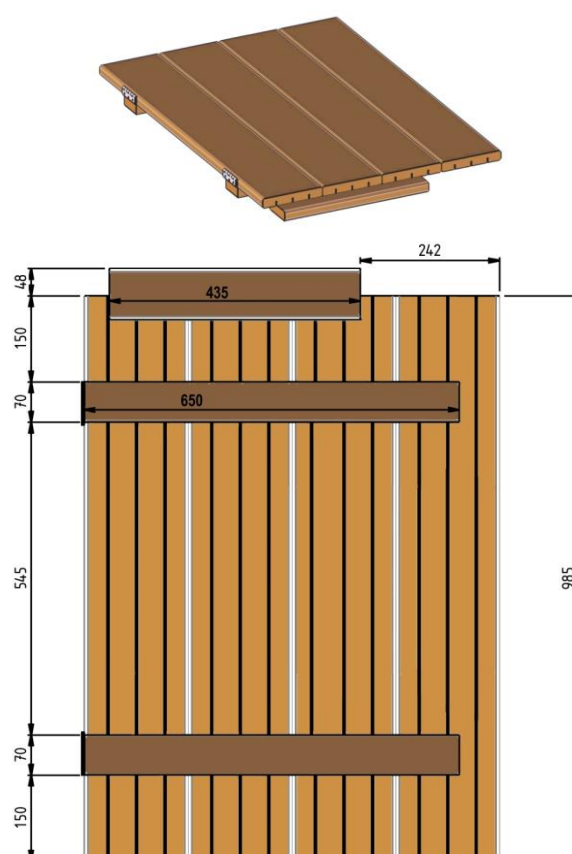
Figure 32 - Assemblage des caillebotis
