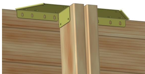
Figure 18 - Mise en place des équerres de margelles en haut des jambes de force
