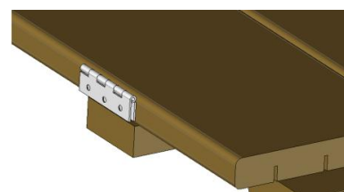
Figure 33 – Mise en place des charnières sur les caillebotis
