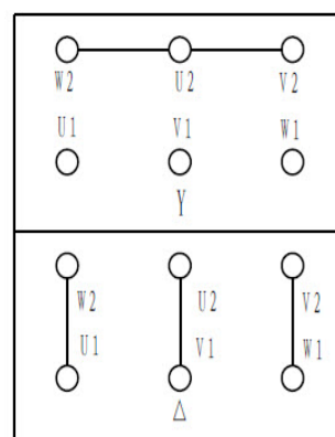
Driefasige aansluiting
