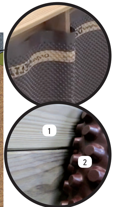
1- Armazón de composite 2- Rollo de protección y de drenaje alveolar de PEHD
