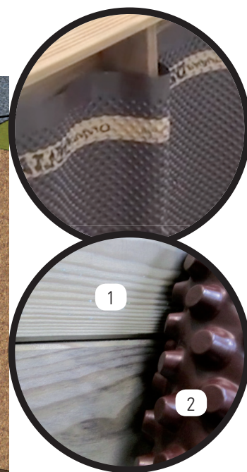
1- Ossature composite 2- Rouleau de protection et de drainage alvéolaire en PEHD
