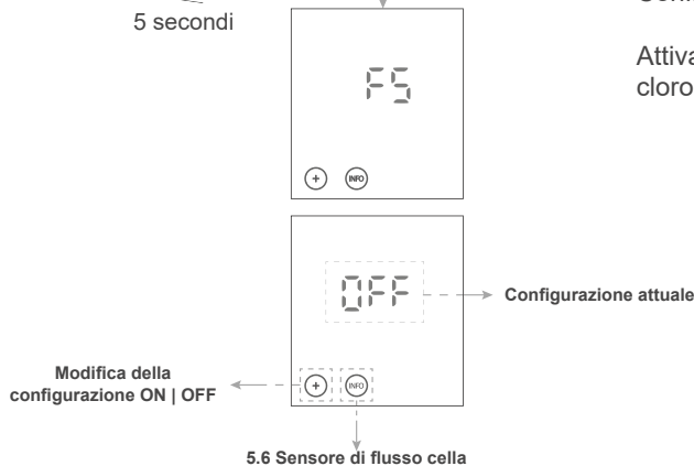
5.6 Sensore di flusso cella
