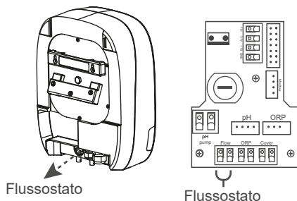
5.6 Sensore di flusso cella
