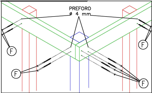
2. fissaggio pali/banchine
