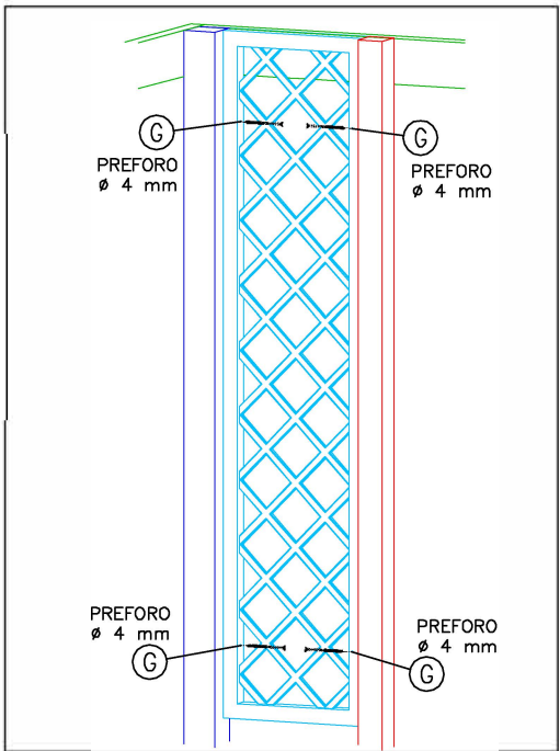
5. fissaggio grigliati
