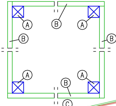
01. schema posizionamento banchine (vista dall'alto)
