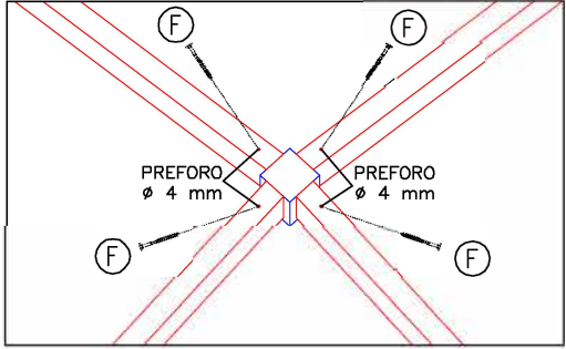
5. fissaggio grigliati
