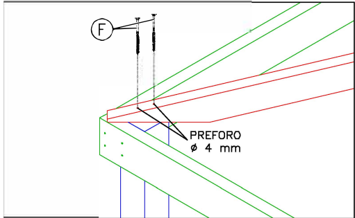
4. fissaggio diagonali/monaco
