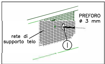
6. fissaggio telo PVC
