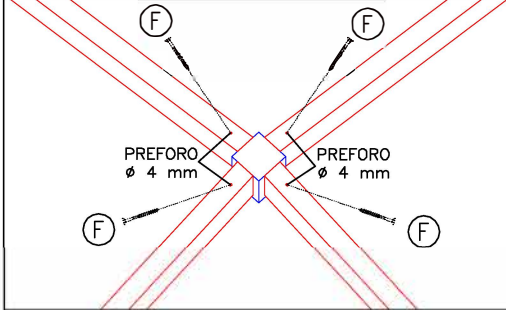
5. fissaggio saette
