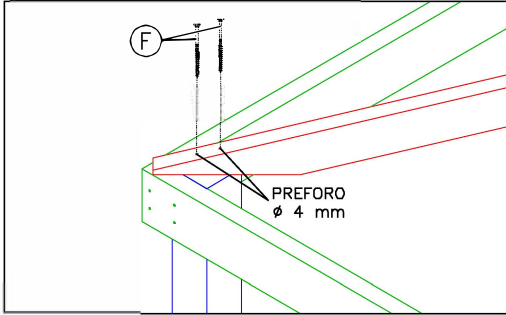
4. fissaggio diagonali/monaco
