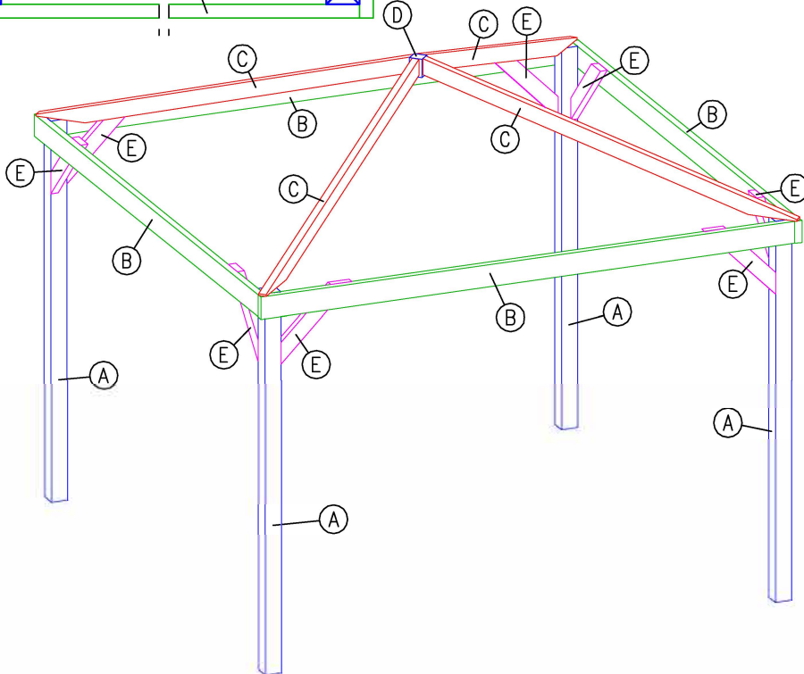
5. fissaggio saette
