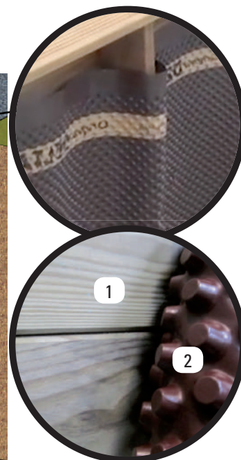
1- Armazón de composite 2- Rollo de protección y de drenaje alveolar de PEHD
